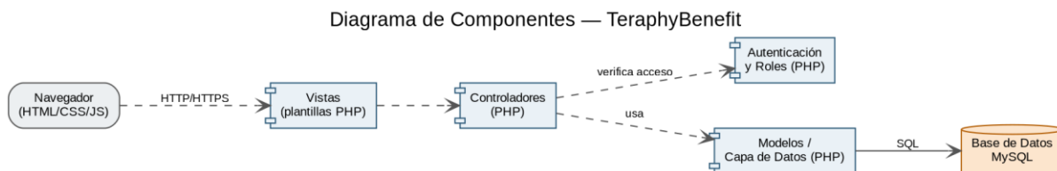
Figura 9. Diagrama de componentes.
